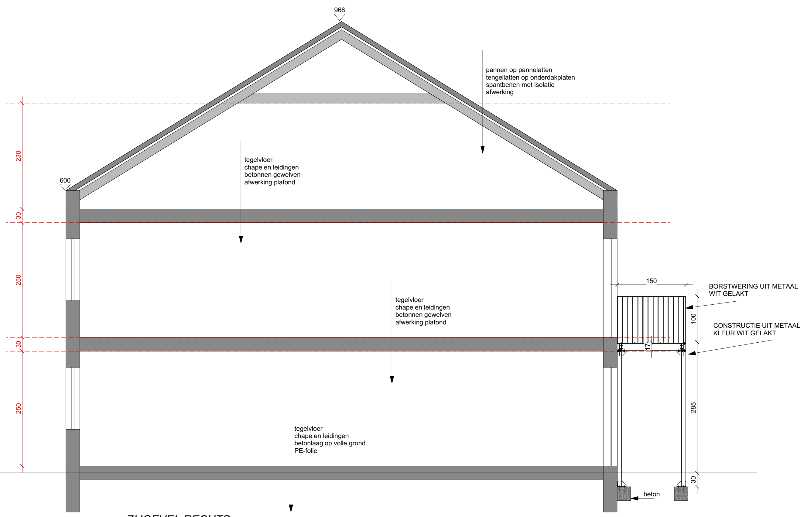
ZIJGEVEL RECHTS schaal 1/50
