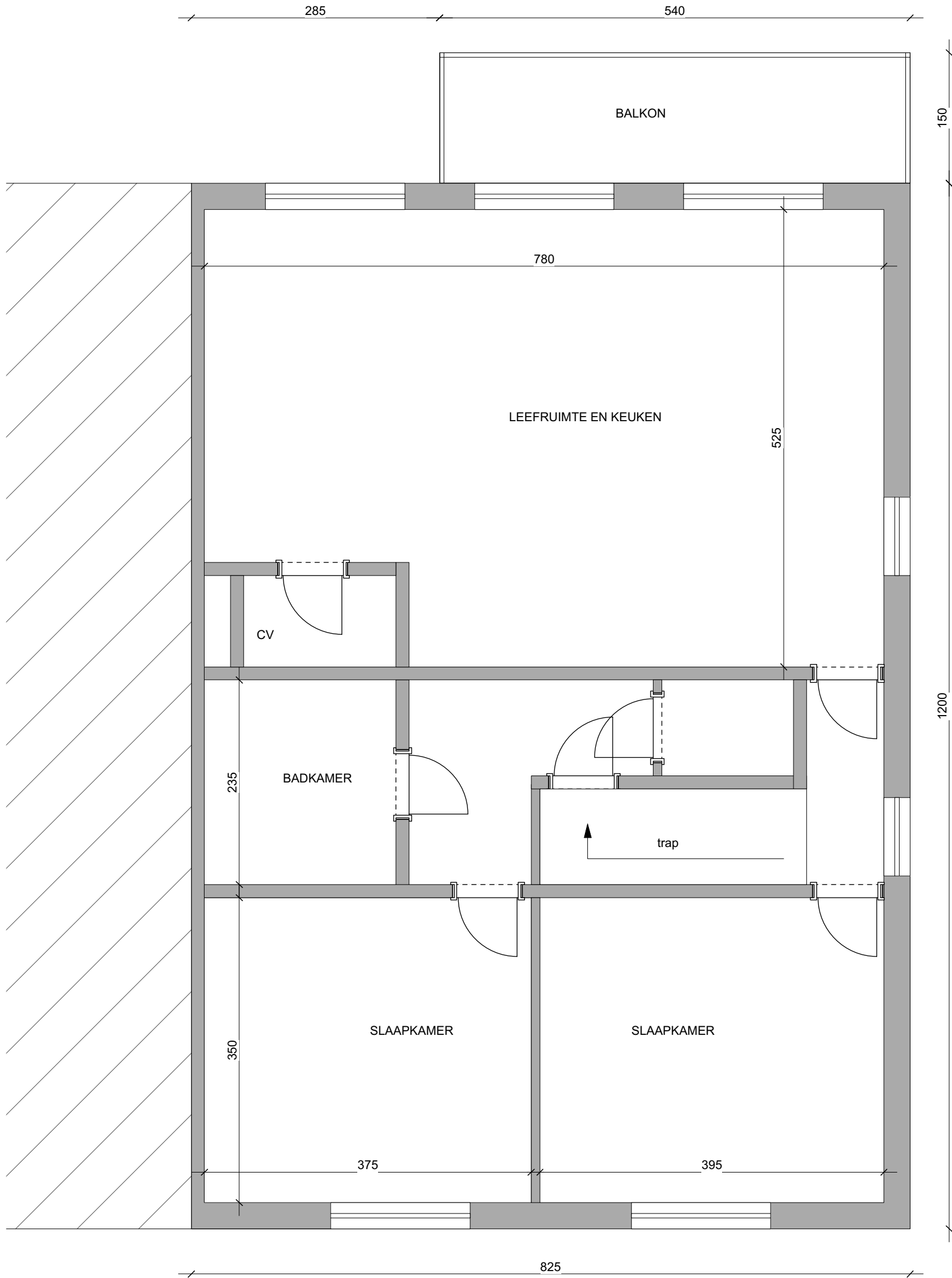
PLAN VERDIEP schaal 1/50
