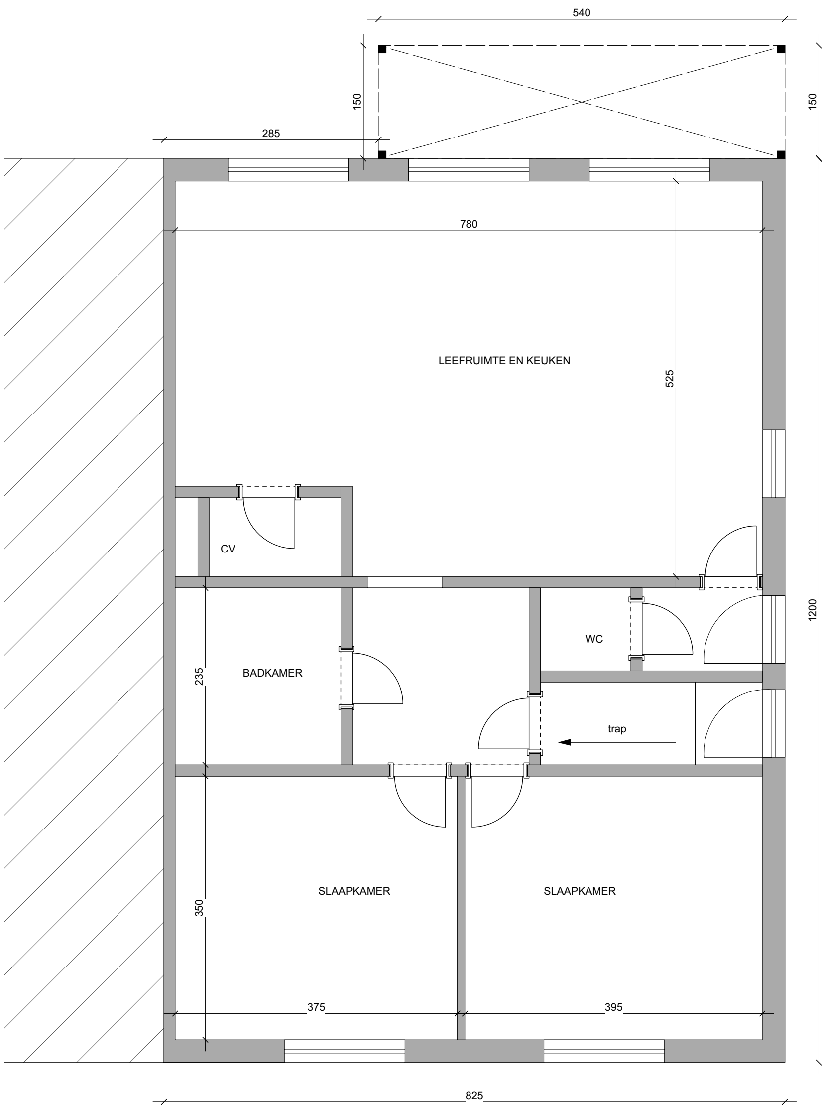
PLAN GELIJKVLOERS schaal 1/50
