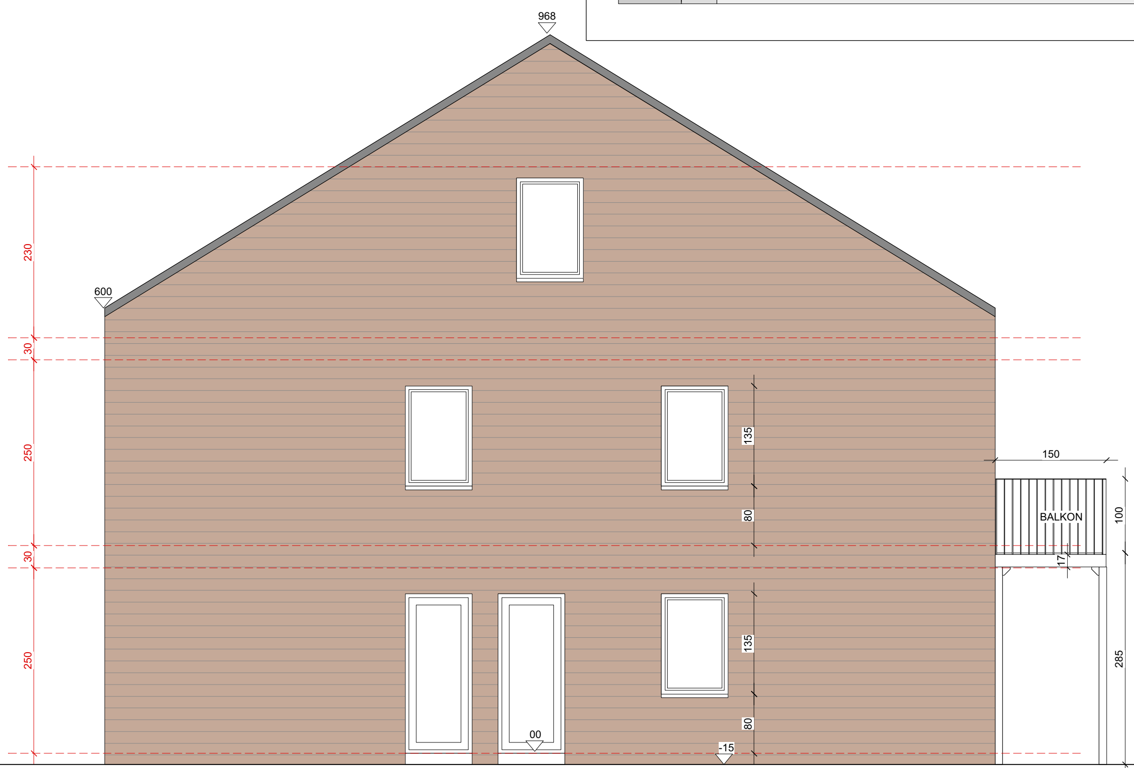
ZIJGEVEL RECHTS schaal 1/50
