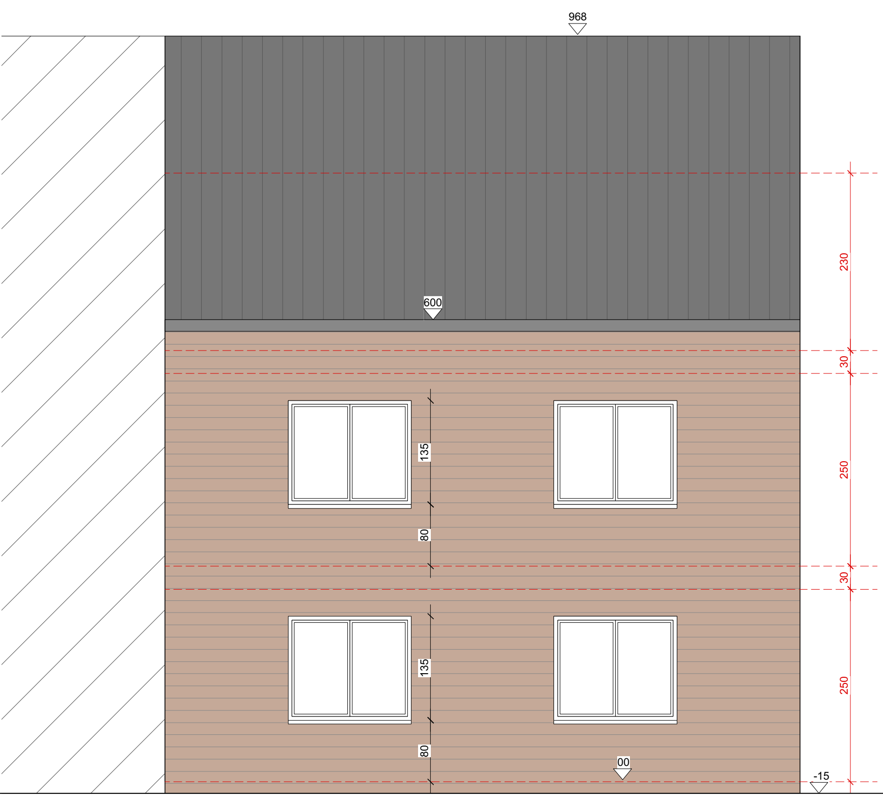
VOORGEVEL schaal 1/50
